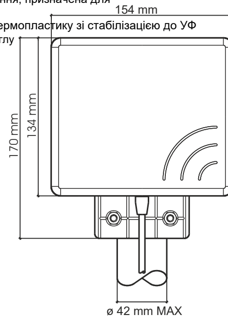
Монтаж на щоглу
